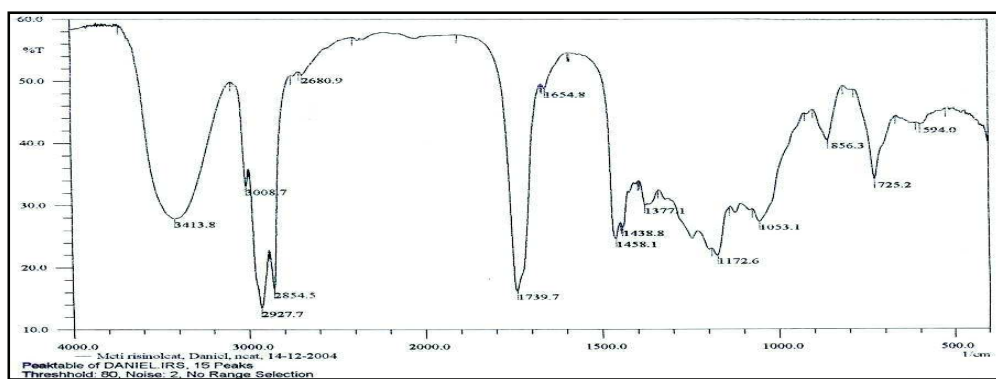
Gambar 2: Spektrum FT-IR senyawa Metil Risinoleat
